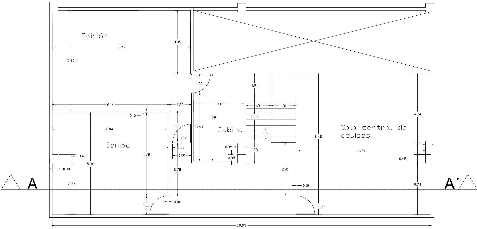
PLANTA MEZZANINE DIMENSIONADA Esc. 1:100
